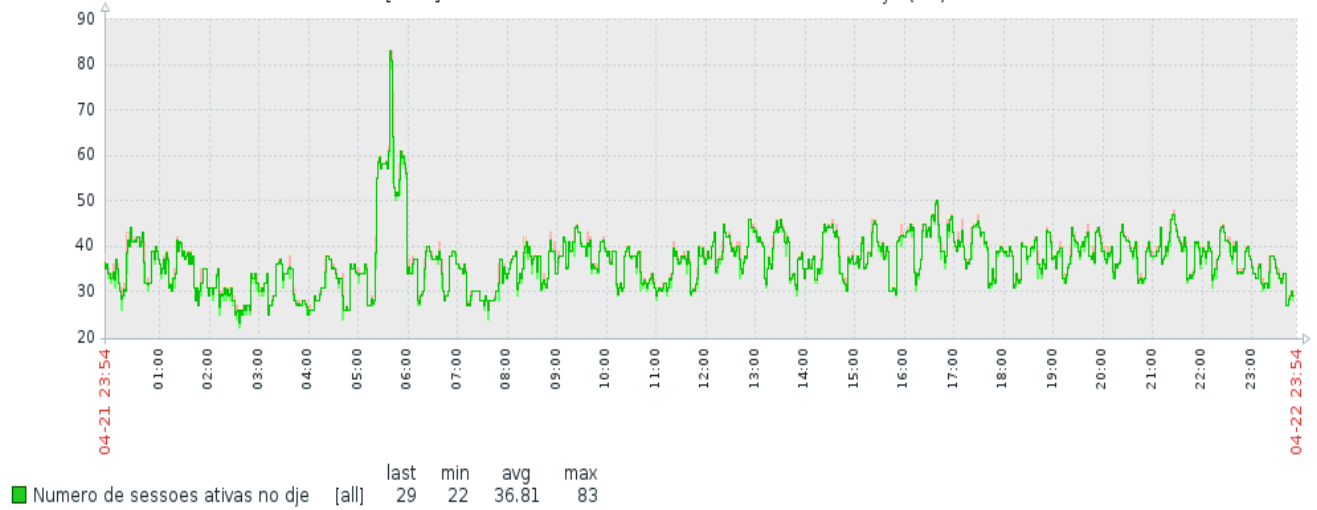
[OL7] Tomcat - 08: Numero de sessoes ativas no dje (1d)
