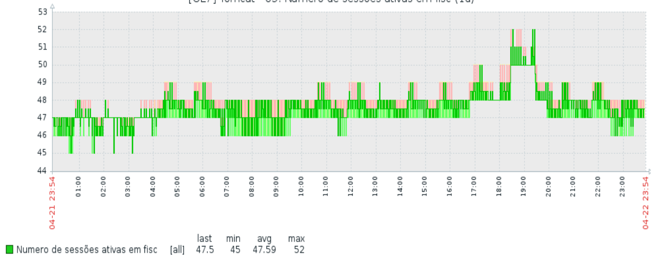
[OL7] Tomcat - 09: Numero de sessões ativas em fisc (1d)
