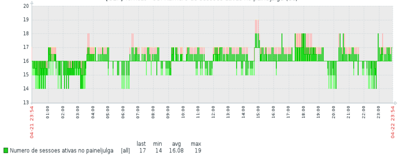
[OL7] Tomcat - 08: Numero de sessoes ativas no paineljuga (1d)
