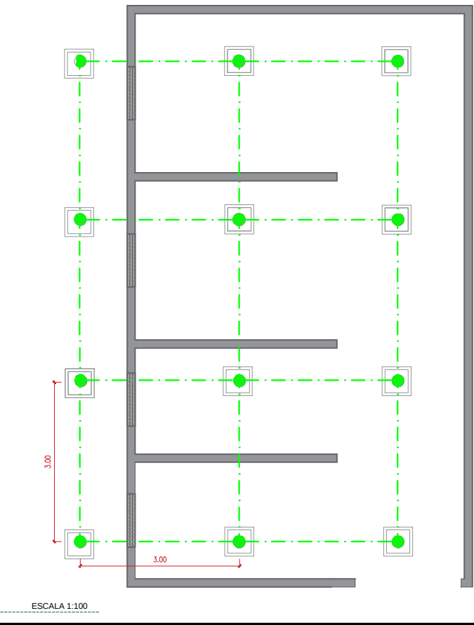
DETALHE - 1 - MALHA DE ATERRAMENTO
