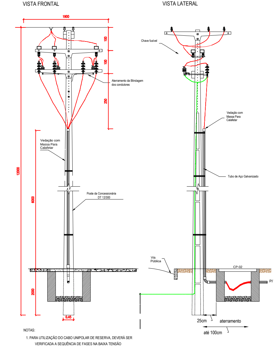
DETALHE ENTRADA-MUFLAS
